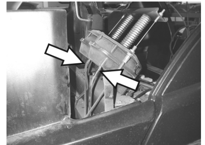
Schlauchanschlüsse zur Unterdruckdose der Kehrwalzenabsenkung
